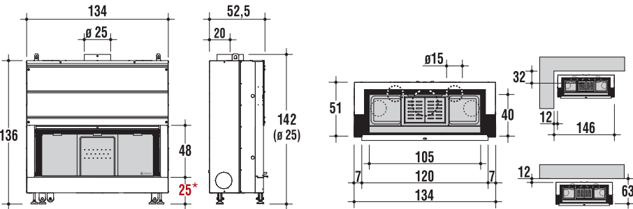
≥ 35* cm hauteur sole foyer LIGHT 06N à bois à air chaud convection naturelle
