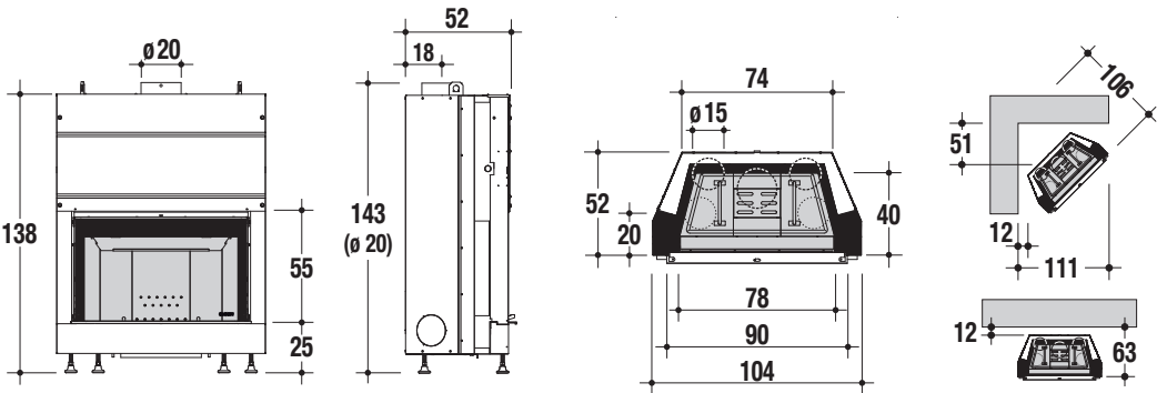
LIGHT O2N S à bois à air chaud convection naturelle
